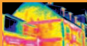
Die Thermographie zeigt deutlich den Wärmeverlust an den rotglühenden Stellen der Hauswand.
